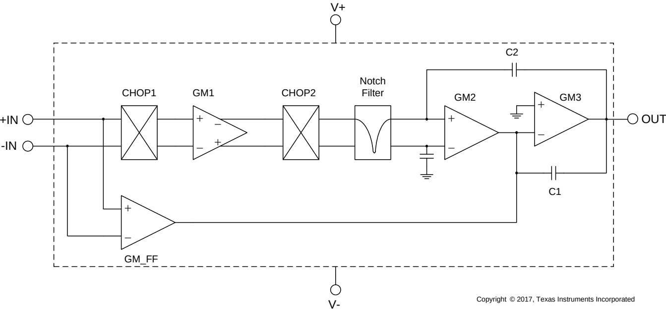
图 37. 功能框图
