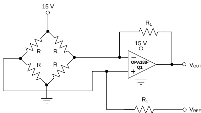
图 46. 桥式放大器
