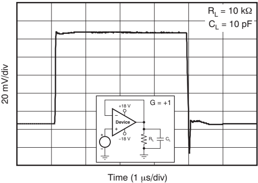
图 27. 正过载恢复
