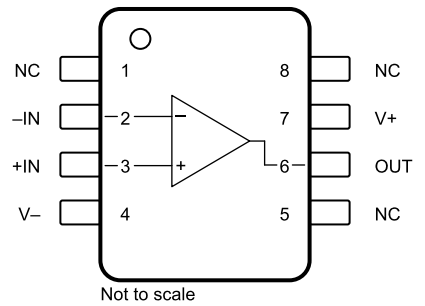
OPA188-Q1 DGK 封装 8 引脚 VSSOP 俯视图
