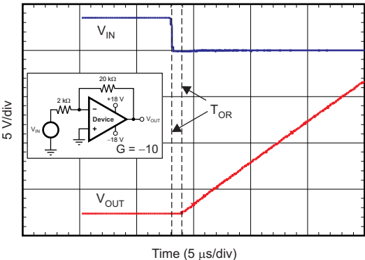
图 26. 无相位反转
