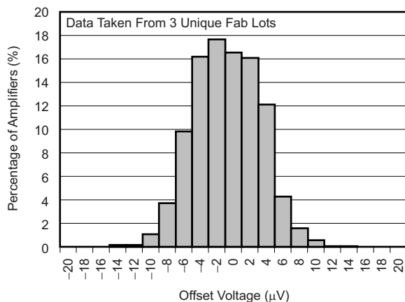
失调电压分布
