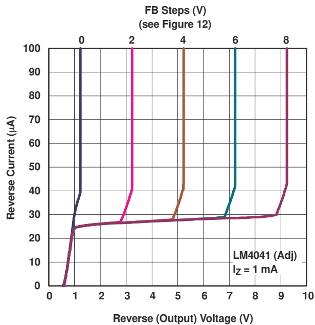
图 13-9. Reverse Characteristics
