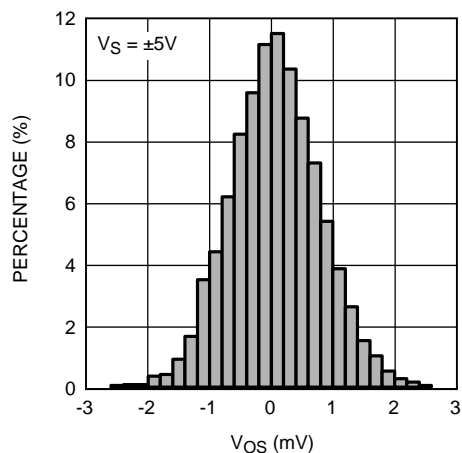
图 7. V_{OS} 分布
