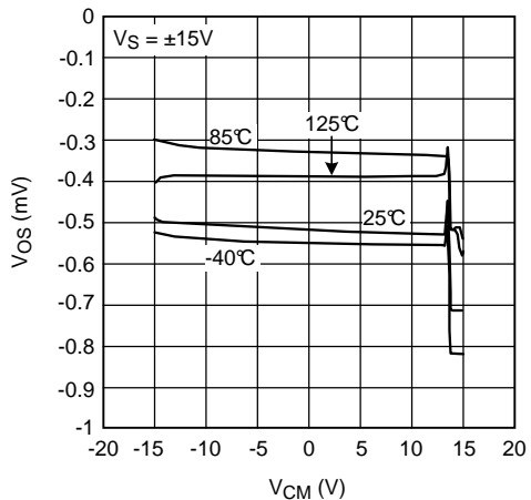
图 15. V_{OS} 与 V_{CM} 间的关系 (单位 2)
