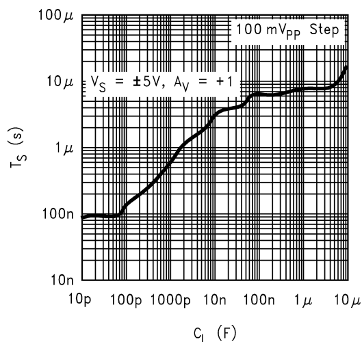
图 61. ±5% 建立时间与容性负载间的关系
