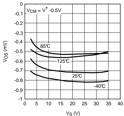
图 21. V_{OS} 与 V_S 间的关系 (单位 2)
