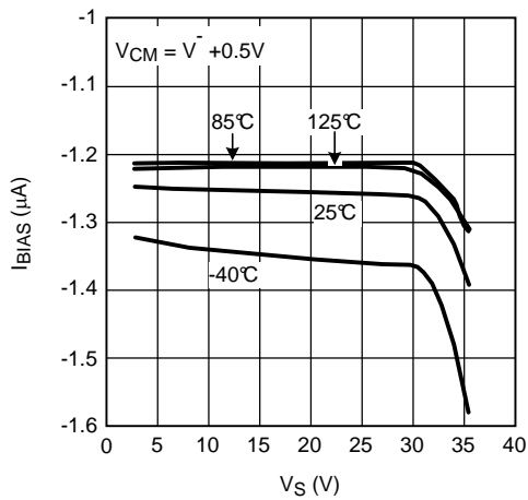
图 26. I_{BIAS} 与 V_S 间的关系
