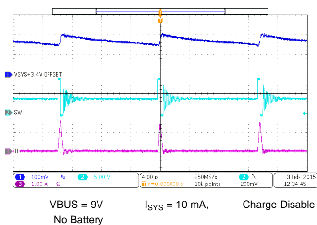
图 55. PFM Switching Waveform
