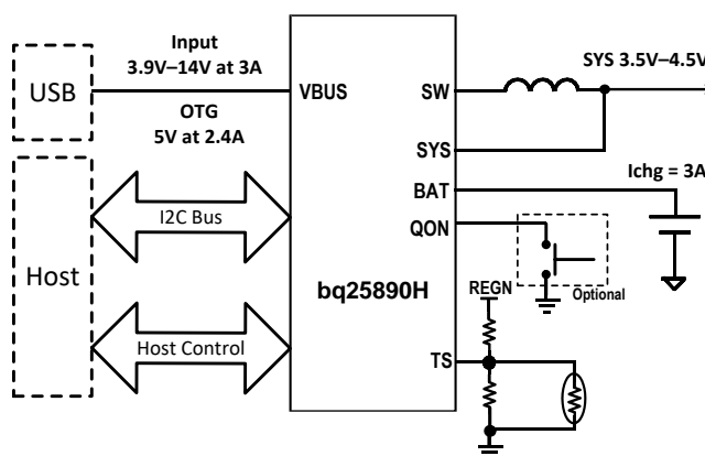
简化原理图
