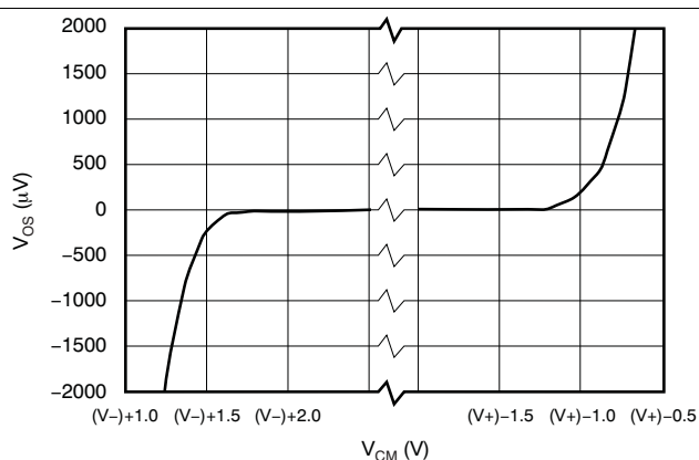
图 14. 失调电压与共模电压间的关系
