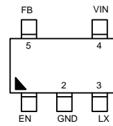
SOT-23-5
