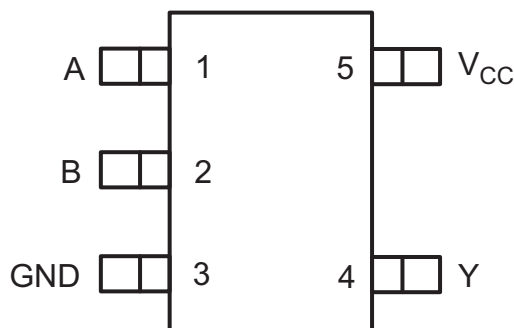
DCK/DBV/DRL 封装 (顶视图)
