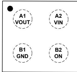
WLCSP-0.8x0.8-4B
