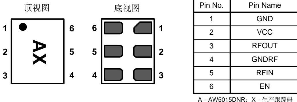
图 1. AW5015 引脚分布及标识图
