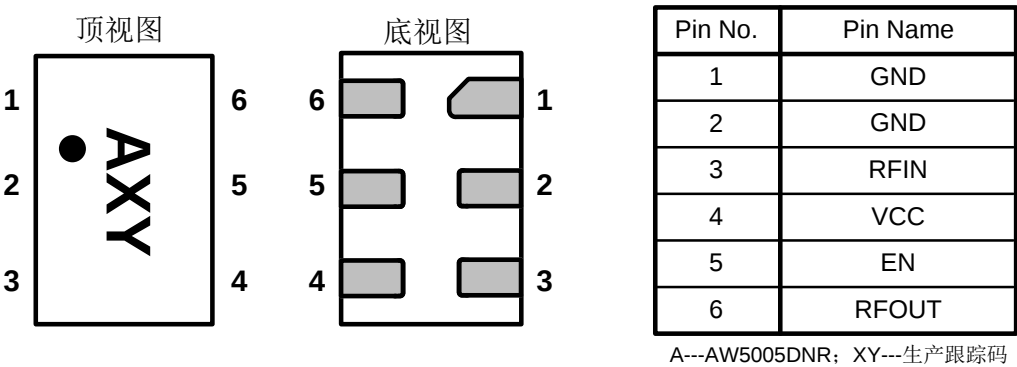
图 1. AW5005 引脚分布及标识图
