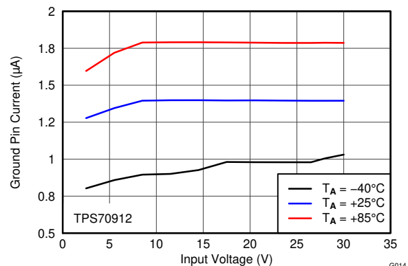
接地电流与 V_{\text{IN}} 和温度间的关系
