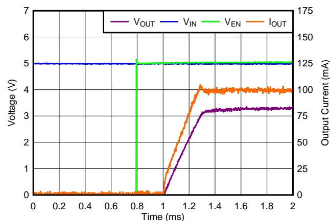
启动波形
